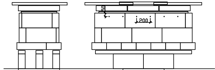
END ELEVATION
